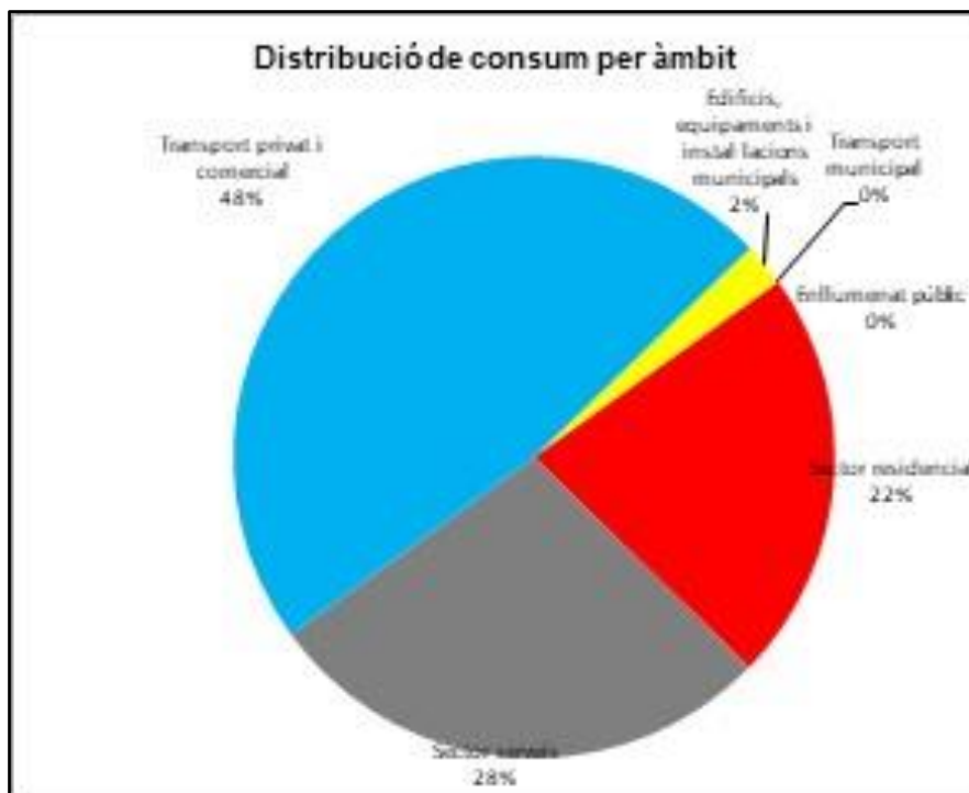
Gràfic 20. Distribució de consums per àmbit (MWh)
