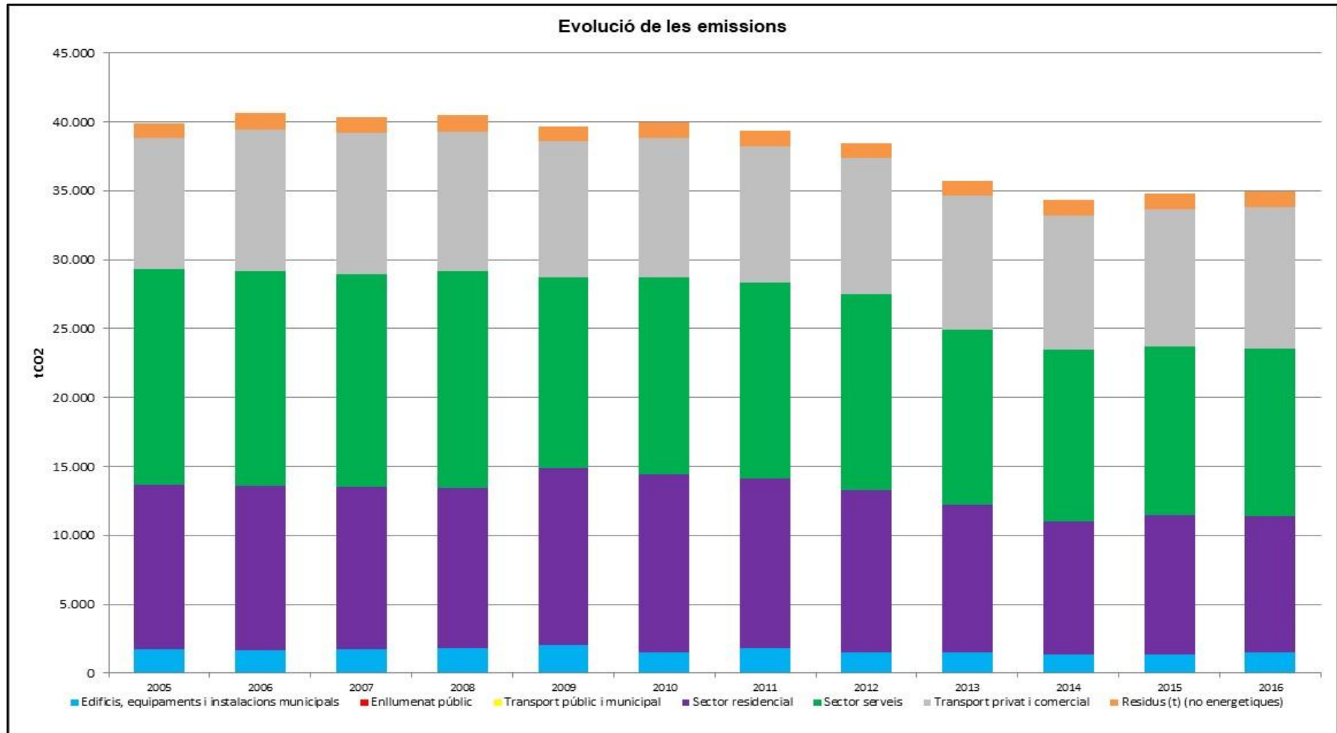
Gràfic 17. Evolució de les emissions totals en el municipi per àmbit (tCO 2 )
