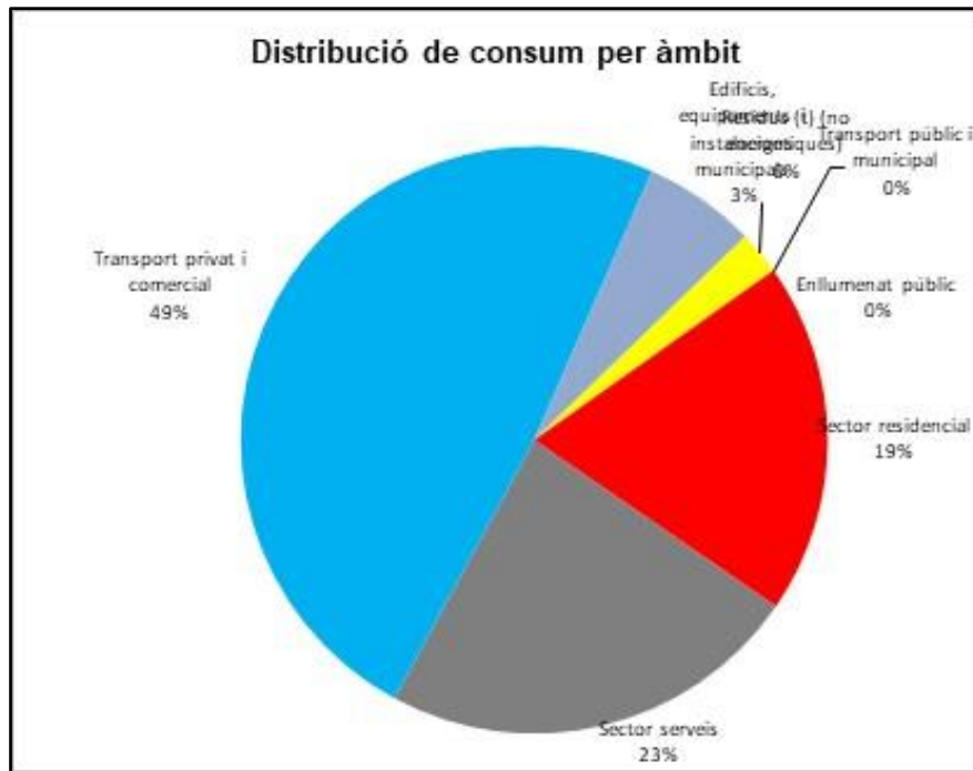
Gràfic 31. Distribució de consums per àmbit (MWh)
