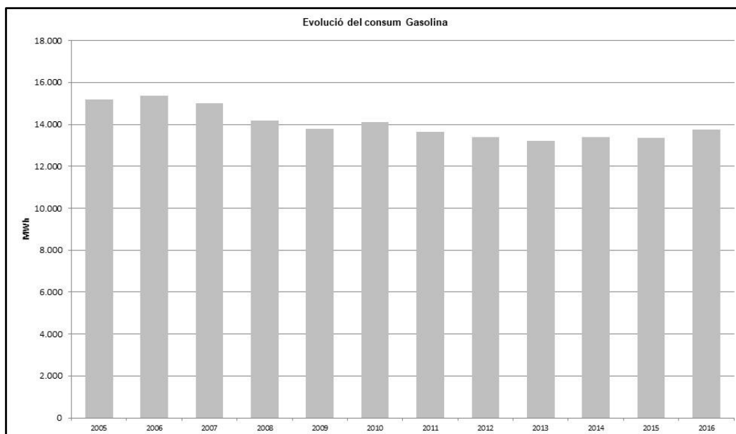
Gràfic 30. Evolució del consum de gasolina (MWh)
