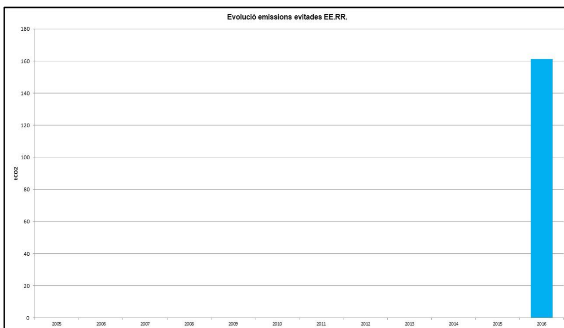
Gràfic 16. Evolució de les emissions evitades mitjançant energies renovables
