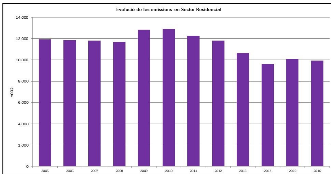
Gràfic 12. Evolució de les emissions del sector residencial
