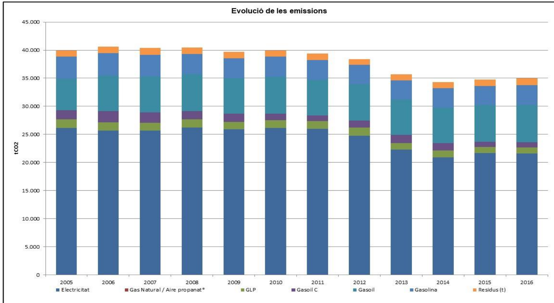
Gràfic 18. Evolució de les emissions totals en el municipi per font (tCO 2 )
