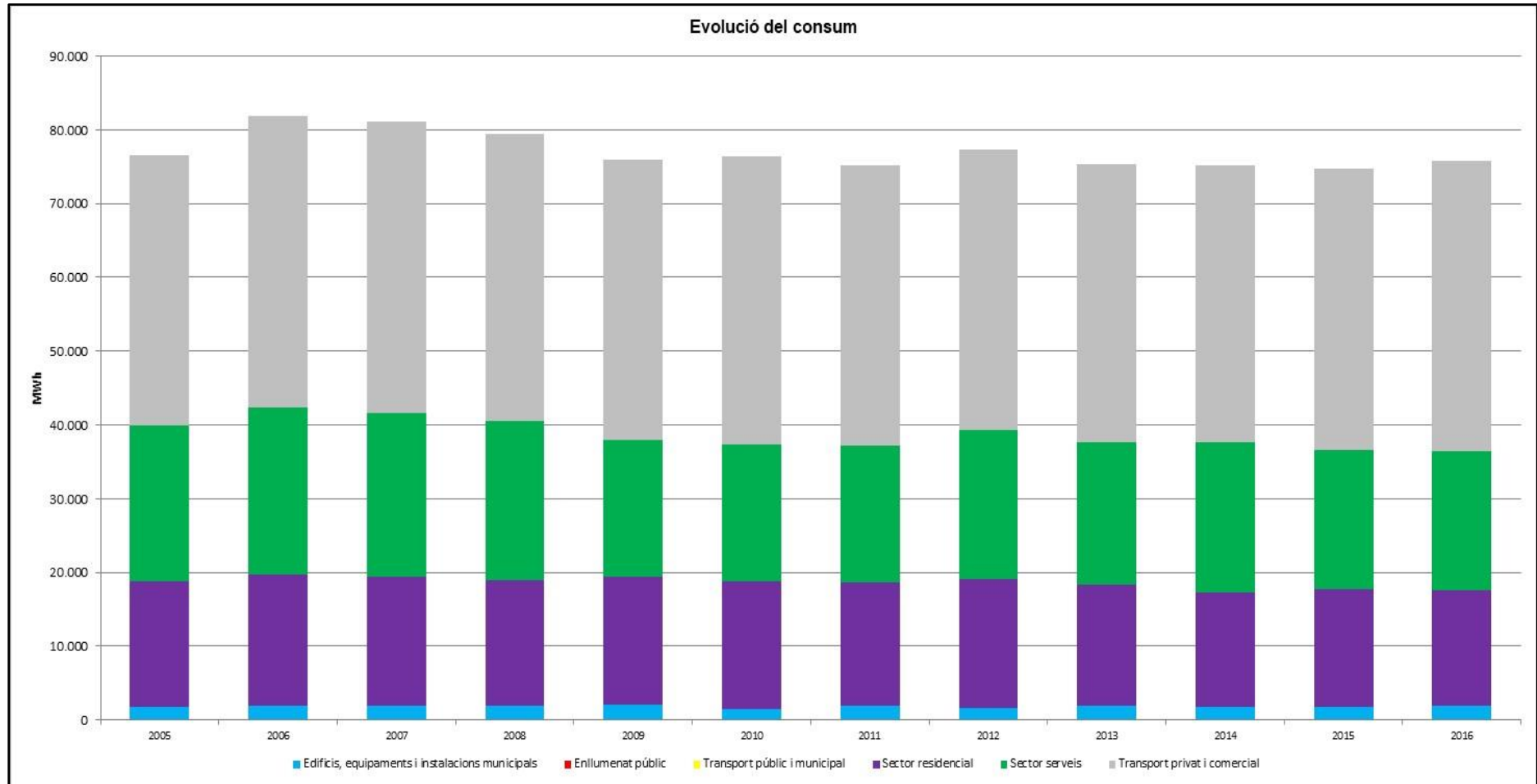
Gràfic 9. Evolució del consum total en el municipi per àmbits (MWh)
